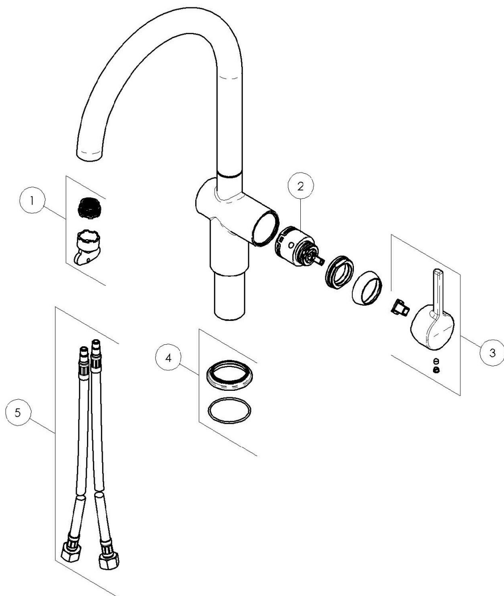
ACTIVE J Swivel Spout 115.0656.874 MB FAJ
