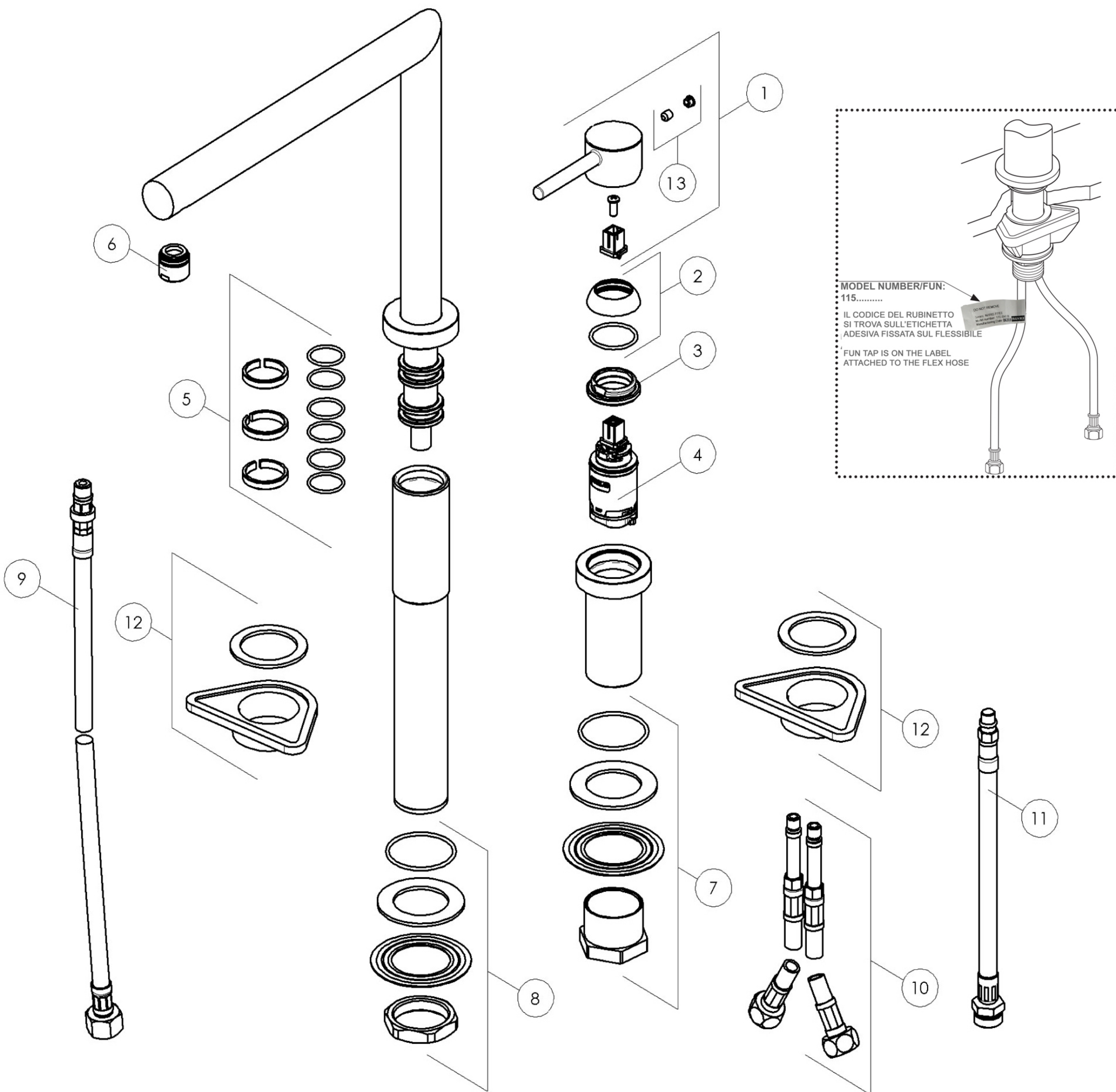
115.0486.980 CROMATO II VERSIONE DIMENSIONI
