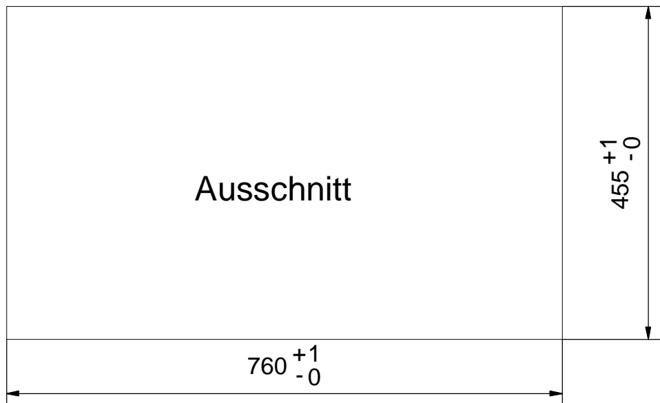
Konstruktionszeichnung 0002-101853
