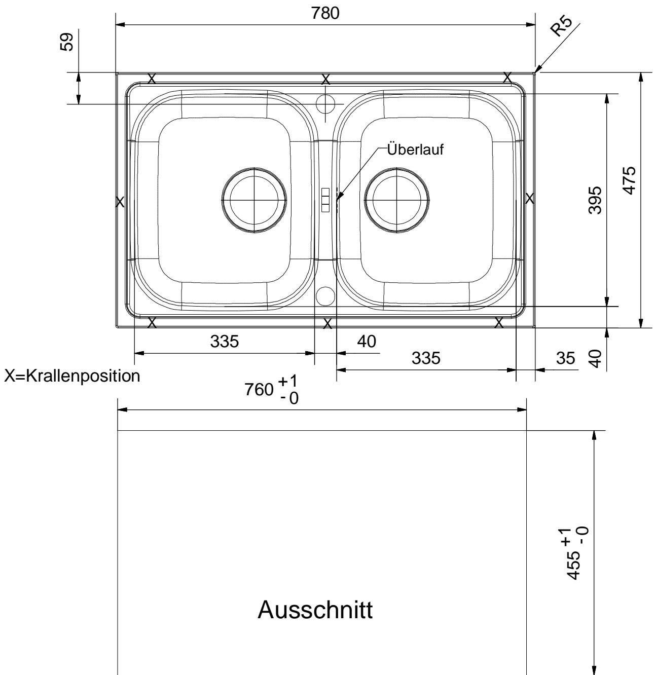
Konstruktionszeichnung 0002-101815
