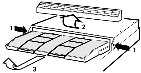
Fig. 9 Trykk inn klipsene på begge sider av ventilatoren (1) og løft løs fronten (2). Dra deretter ut og løft løs filterholderen (3), Fig. 9.
