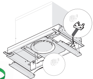
2) إزالة البراغي (M4x10)x4
