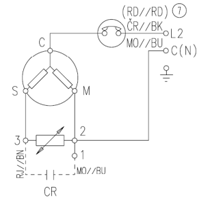
EMBRACO EGZS
