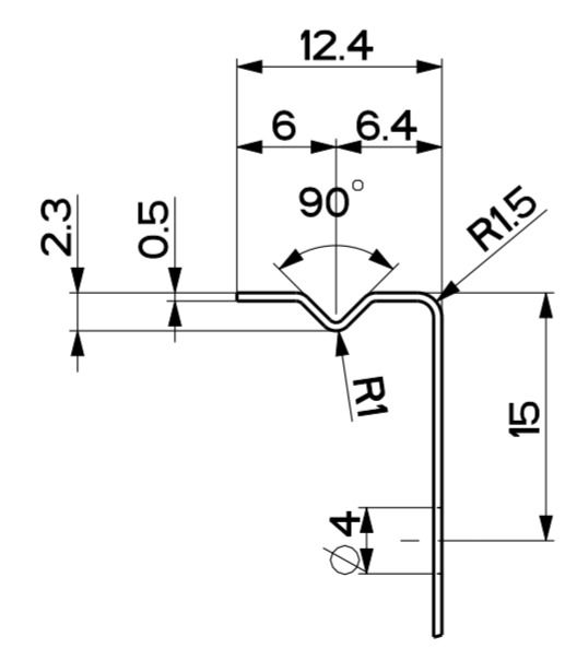
DETTAGLIO A SCALA 2:1
